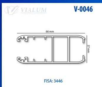
HOJA PUERTA EUROPEA
