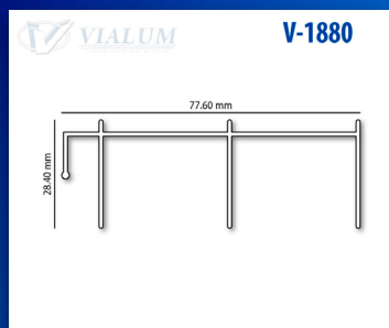
RIEL SUPERIOR PUERTA CORREDIZA ECONÓMICA
