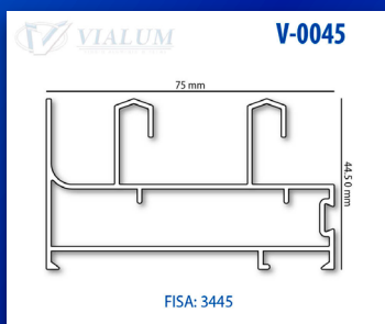
RIEL PUERTA EUROPEA
