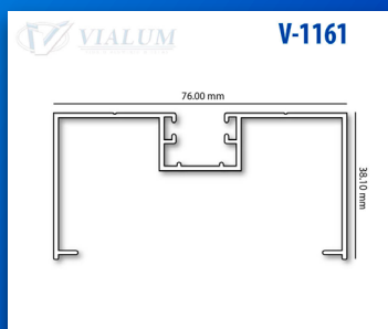
PERIMETRAL FIJO MAMPARA SERIE 200
