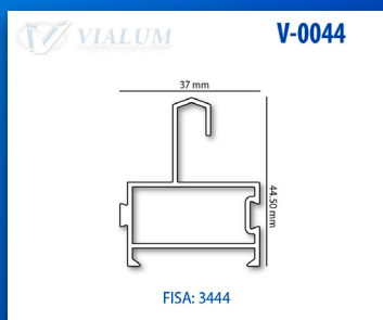
ADAPTADOR DE RIEL PUERTA EUROPEA
