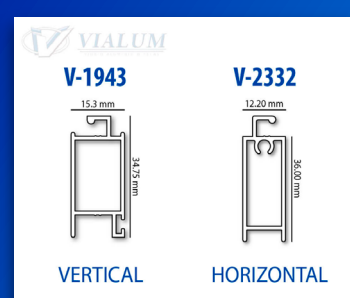
MALLAS PUERTA CORREDIZA ECONÓMICA
