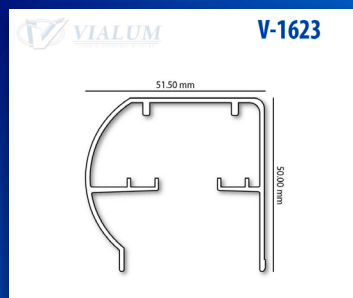
RIEL SUPERIOR PUERTA DE BAÑO ESTANDAR
