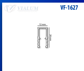
VERTICAL DE HOJA PUERTA DE BAÑO NACIONAL
