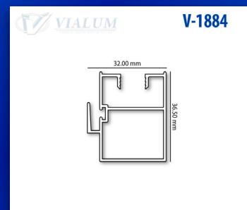
ENTRECIERRE PUERTA CORREDIZA ECONÓMICA
