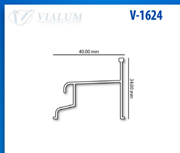
RIEL INFERIOR PUERTA DE BAÑO ESTANDAR
