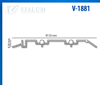
RIEL INFERIOR PUERTA CORREDIZA ECONÓMICA
