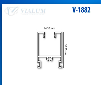
HORIZONTAL SUPERIOR PUERTA CORREDIZA ECONÓMICA
