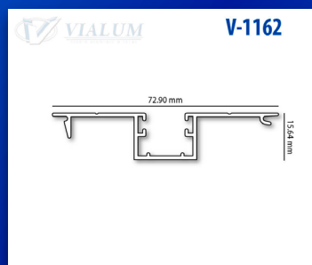
TAPA PERIMETRAL FIJA ACANALADA MAMPARA SERIE 200
