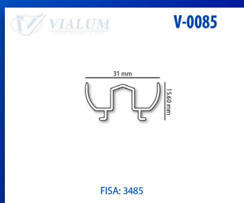
ADAPTADOR PUERTA EUROPEA
