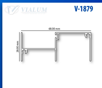
JAMBA MARCO PUERTA CORREDIZA ECONÓMICA
