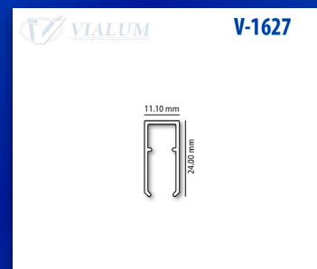
VERTICAL PUERTA DE BAÑO ESTANDAR
