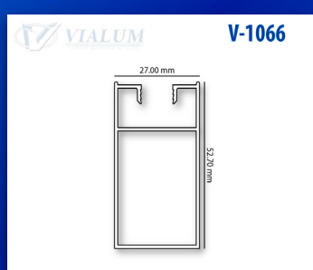
VERTICAL CHAPA PUERTA CORREDIZA ECONÓMICA
