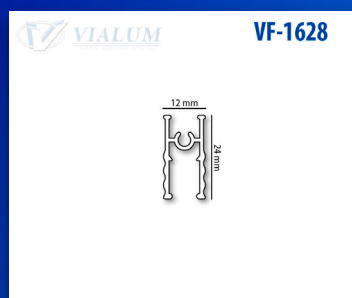
HORIZONTAL DE HOJA INFERIOR PUERTA DE BAÑO NACIONAL
