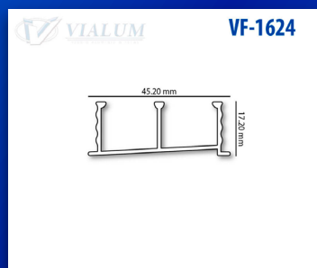
RIEL INFERIOR PUERTA DE BAÑO NACIONAL
