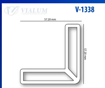
ANCLA PUERTA EUROPEA
