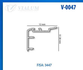
ENTRECIERRE PUERTA EUROPEA
