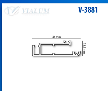
MALLA PUERTA EUROPEA
