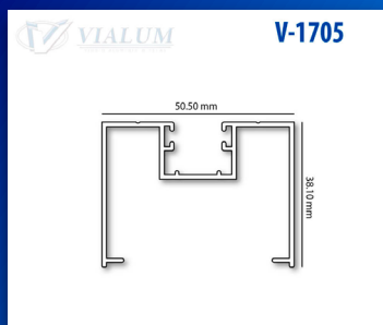
PERIMETRAL FIJO MAMPARA SERIE 100
