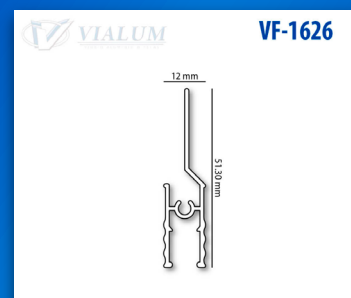
HORIZONTAL DE HOJA SUPERIOR PUERTA DE BAÑO NACIONAL
