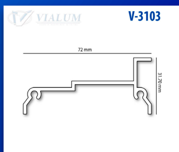
ANCLA MAMPARA SERIE 200
