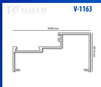
PERIMETRAL MÓVIL MAMPARA SERIE 200
